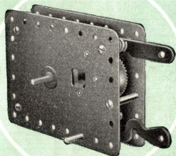
Moteur mécanique No. 1 Veer-motor No. 1
